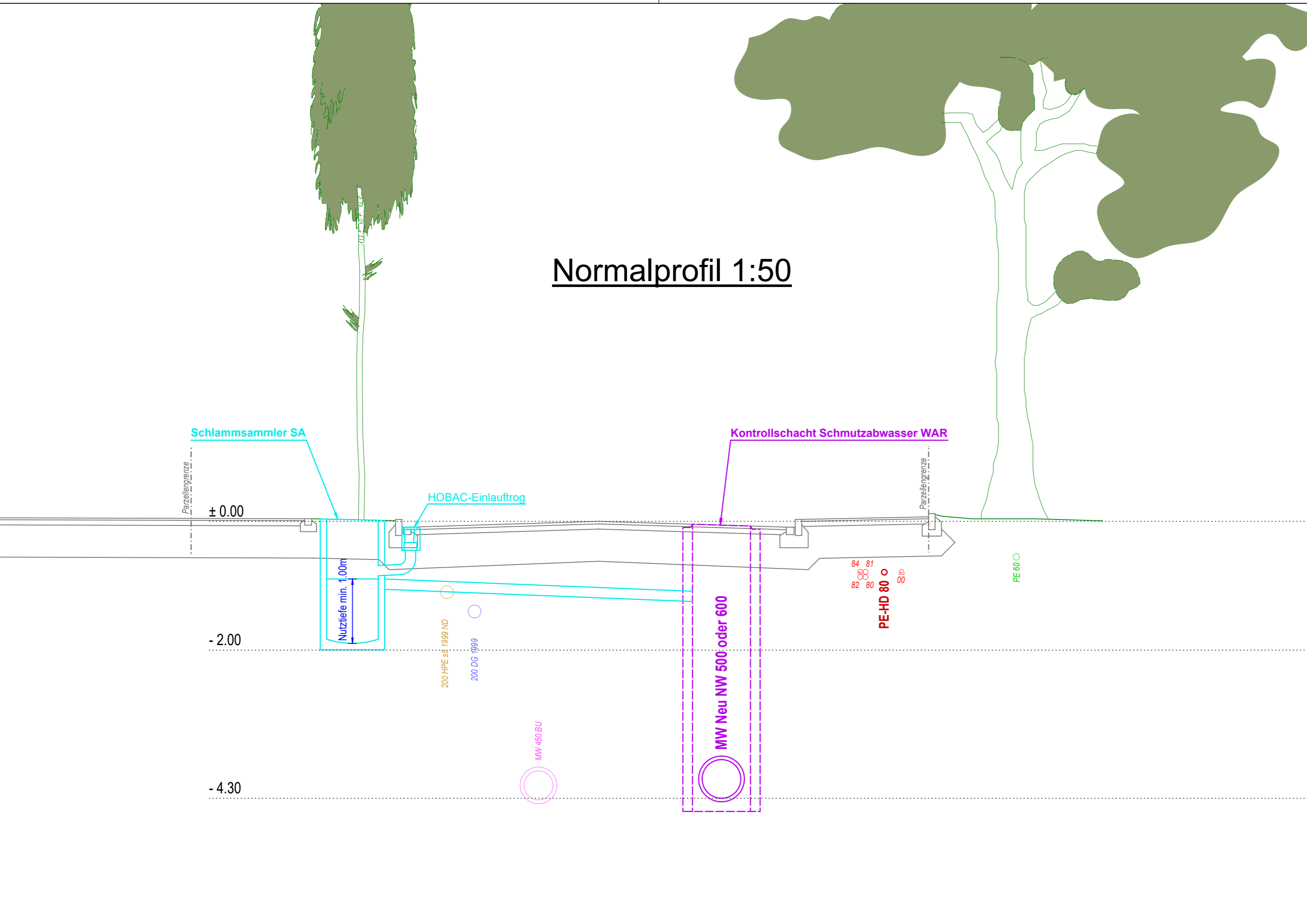
Normalprofil 1:50
