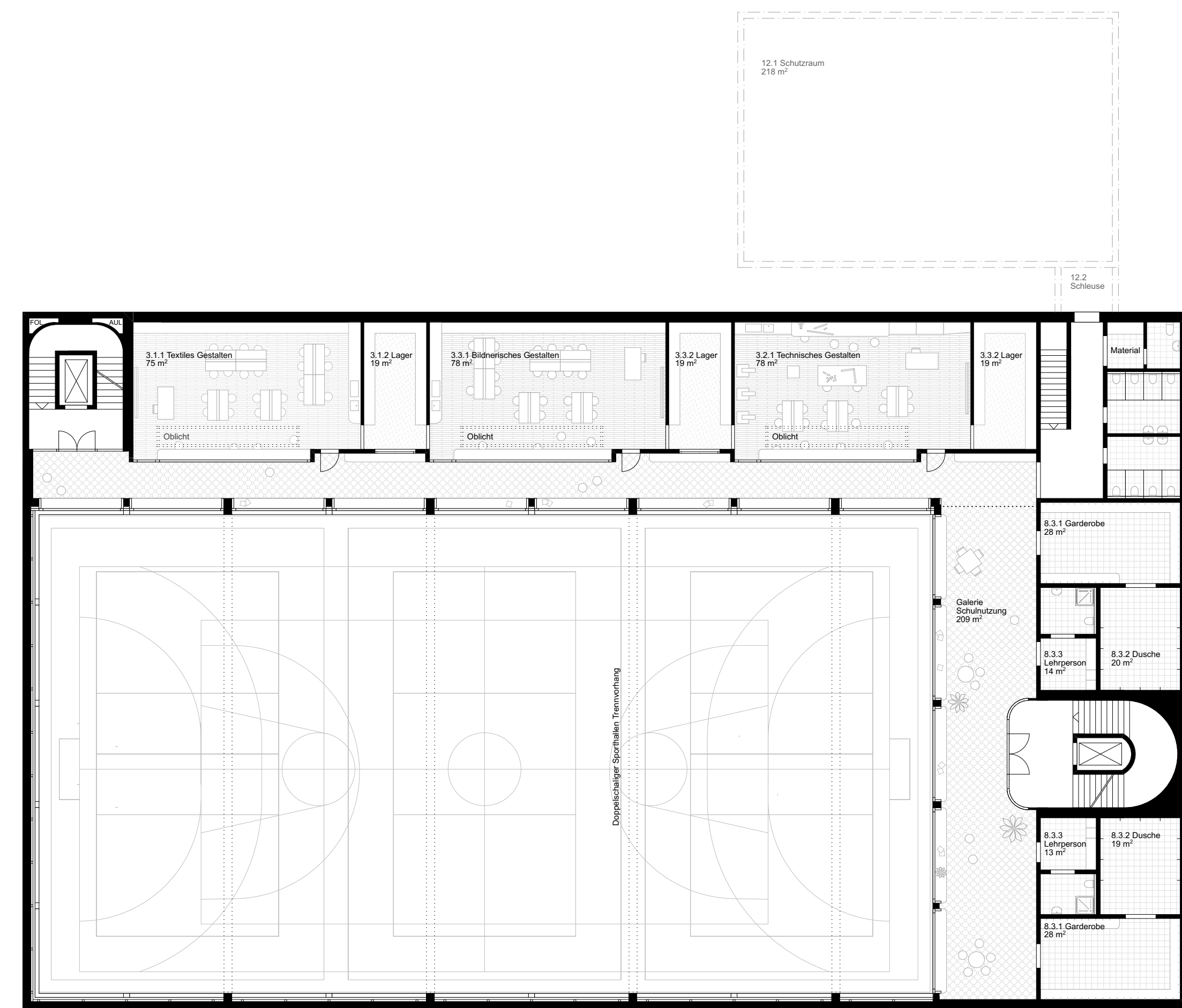
Grundriss 1. Untergeschoss Sporthalle 1:200
