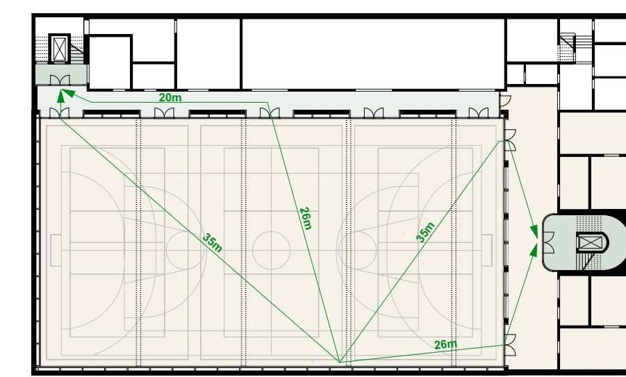
Fluchtwegkonzept
