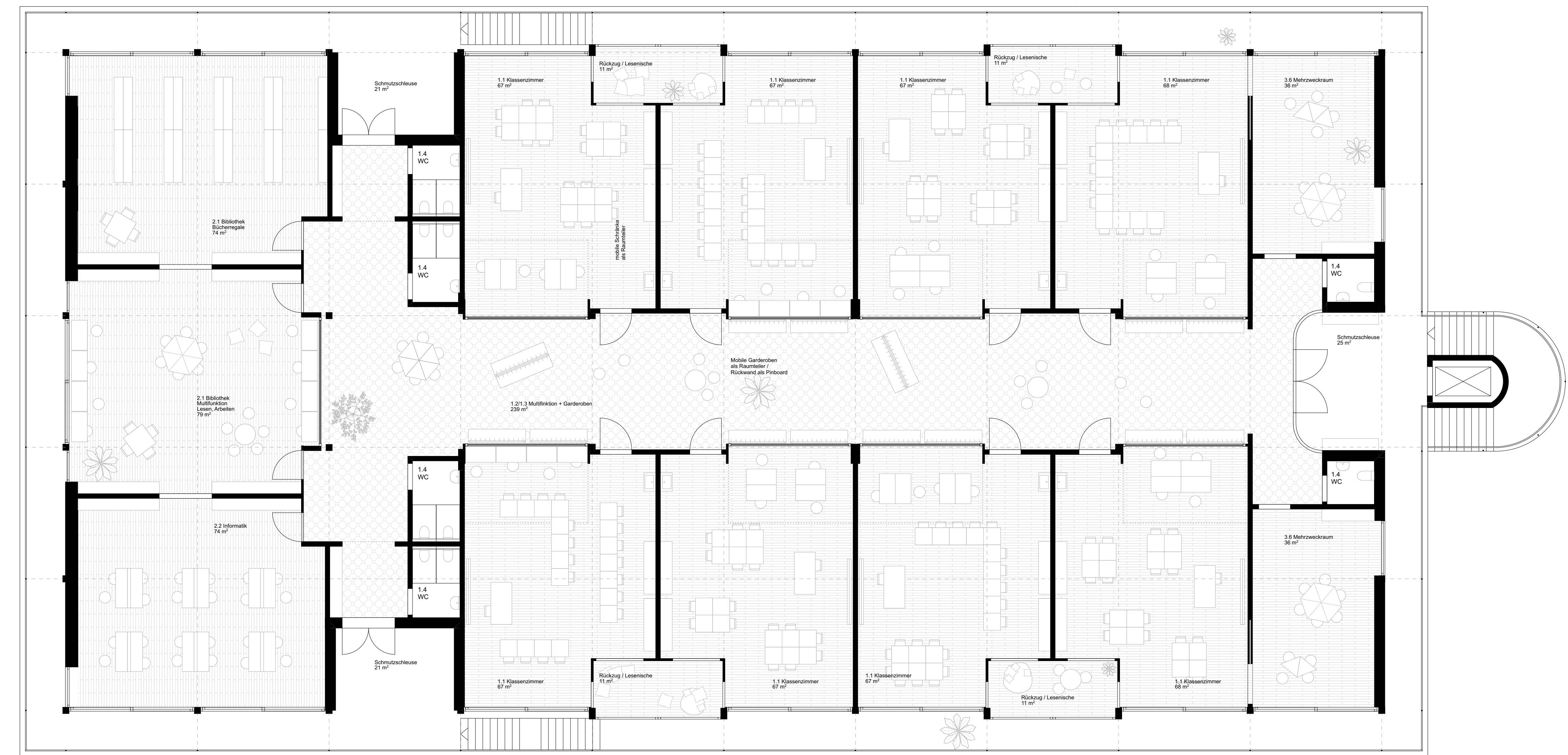
Grundriss 2. Untergeschoss Primarschule mit Sporthalle 1:100
