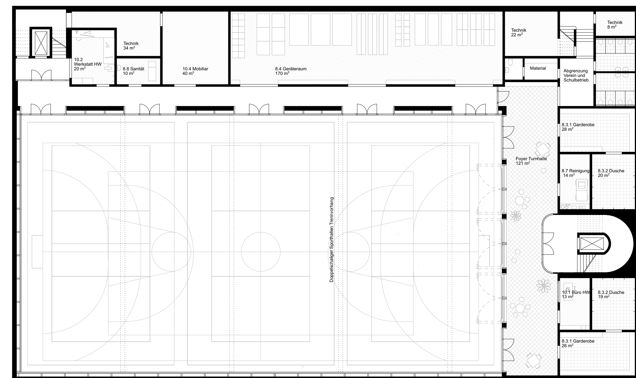
Grundriss 2. Untergeschoss Sporthalle 1:200
