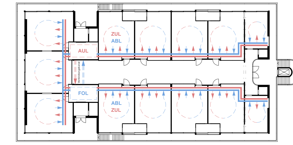
Lüftungskonzept
